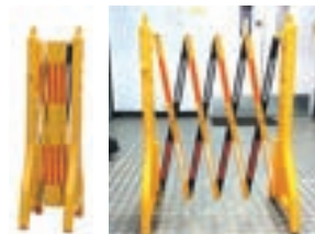
AP1400 注水式塑料伸縮反光圍欄 縮合: 34cm / 展開: 2.5米 96cm(H) · 3kg
