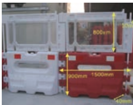
CY03B 水馬 900(H)x1500(L)x400(D)mm 顏色：紅/白色 配白色磨砂面屏風 可配水馬套(可絲印公司Logo)
