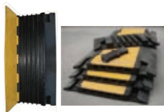
橡膠臨時電線槽 安裝, 拆遷簡易, 堅固耐用 分別有二線 / 三線 / 五線可供選擇
